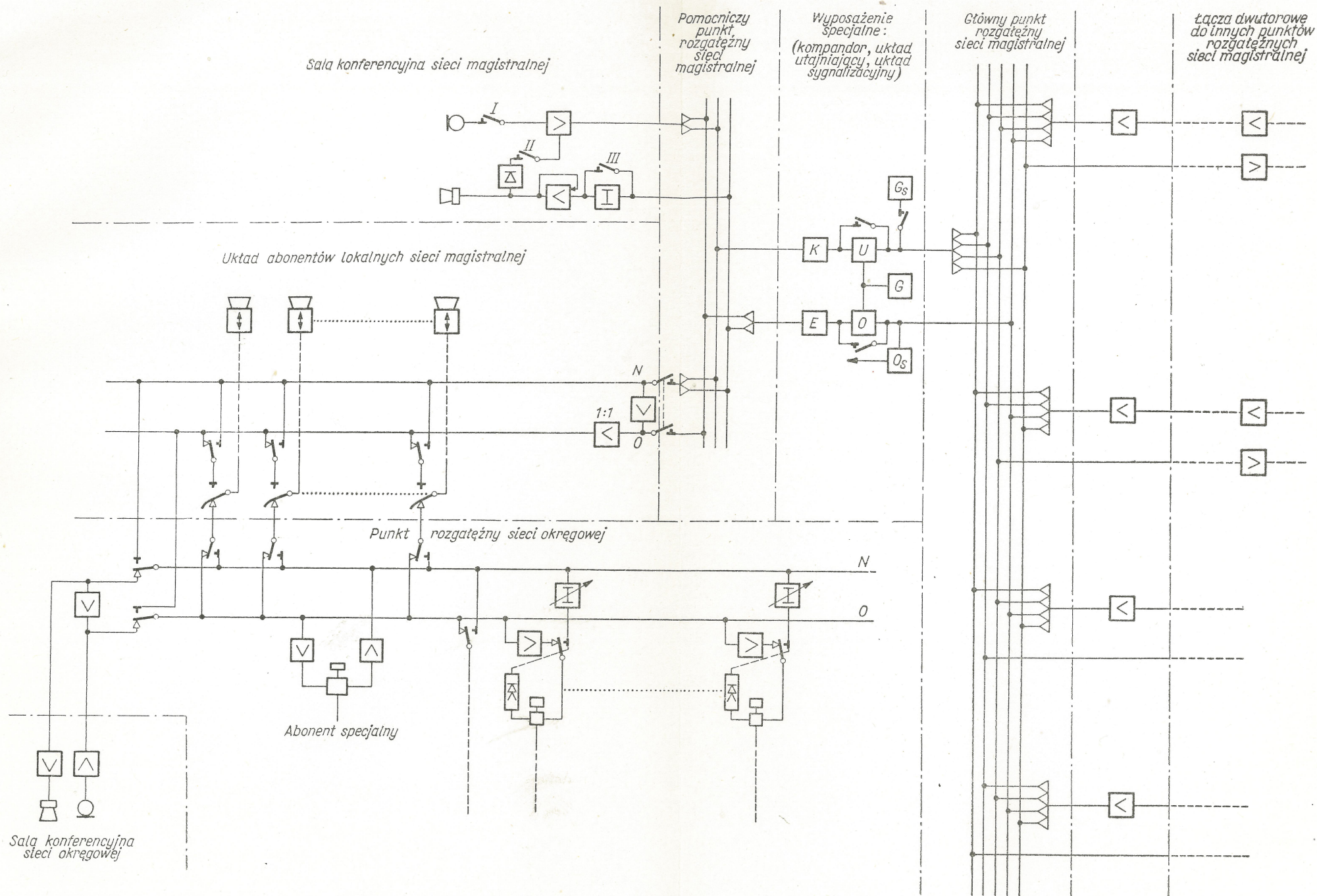
Rys. 2. Schemat współpracy sieci magistralnej z siecią okręgową
